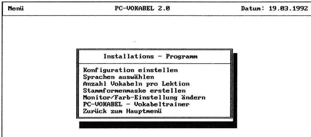
Abb. 3.4: Das Installations-Menü
