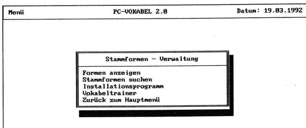
Abb. 3.3: Das Stammformen-Menü
