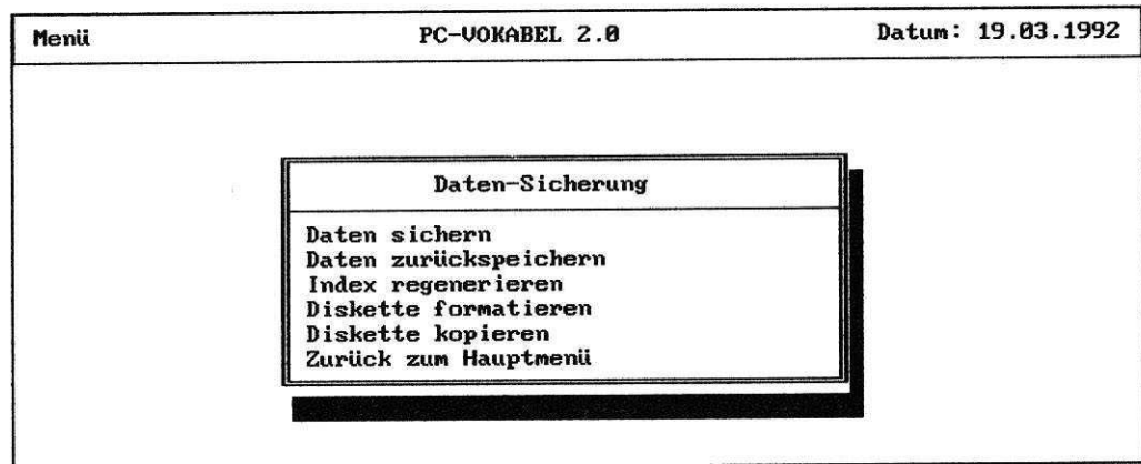
Abb. 3.7: Das Datensicherungs-Menü
