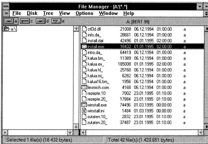
Abb. 1.4: Nach einem Doppelklick auf „install.exe“...
